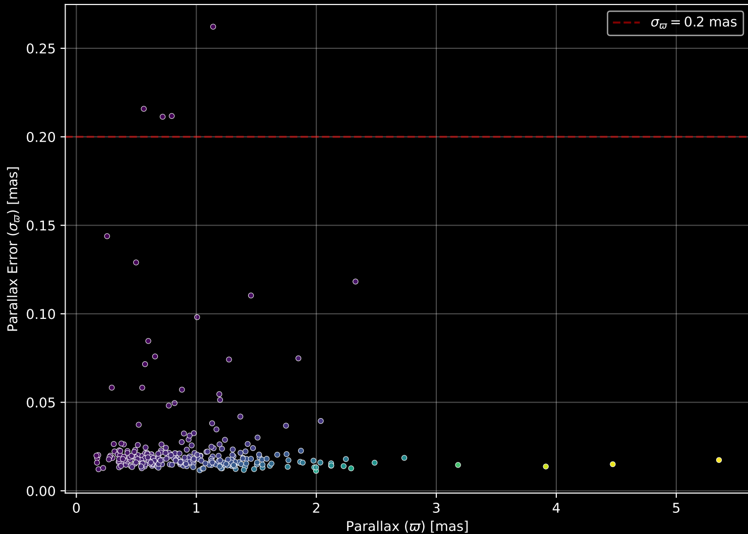
GALAH DR4 Field: [9274] Parallax Quality (n= 270)
