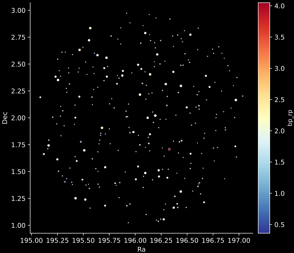
GALAH DR4 Field: [9274] Stars: 270
