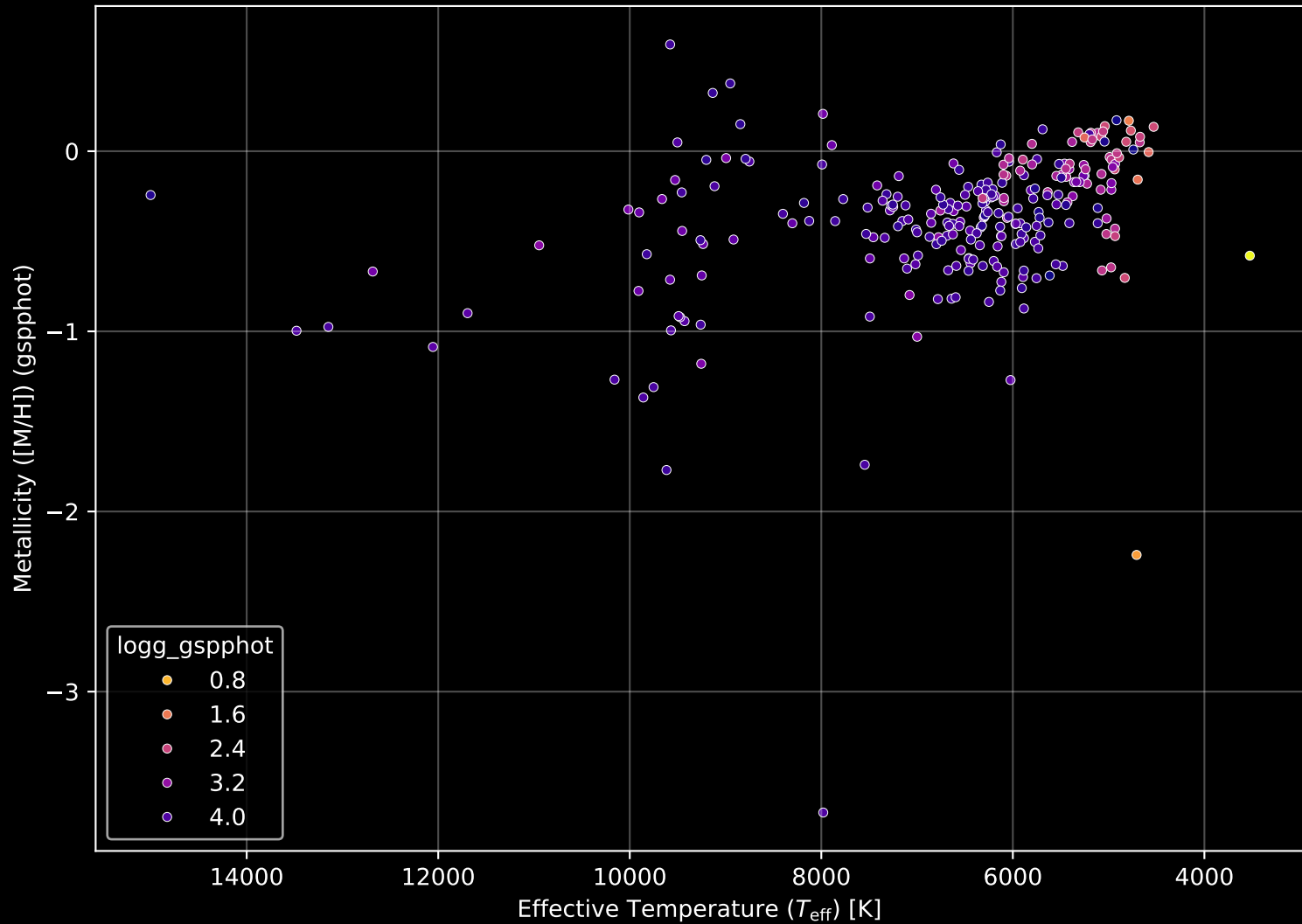
GALAH DR4 Field: [9274] Stellar Population Parameters (n= 270)
