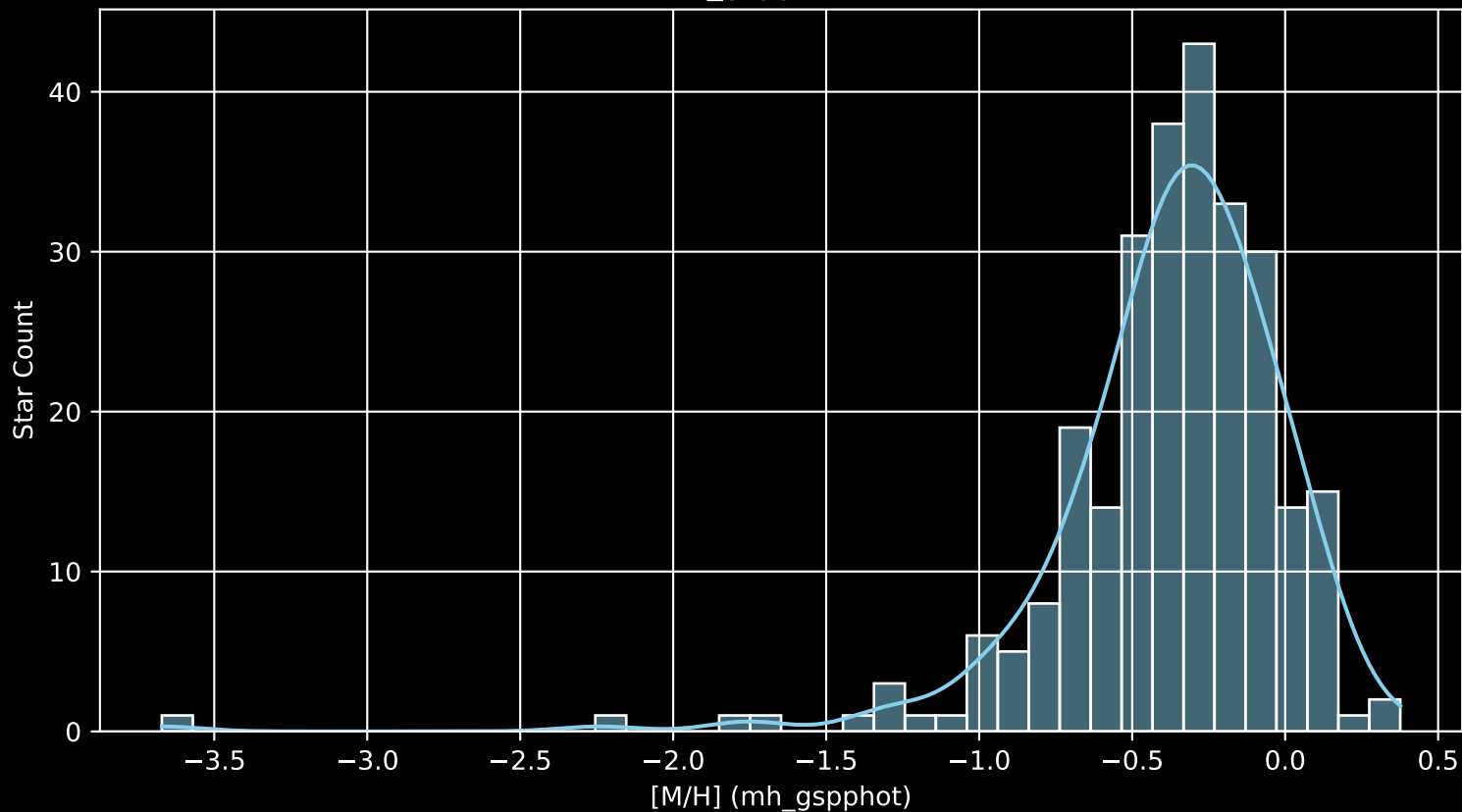
GALAH DR4 Field: [9274] [M/H] (mh_gspphot) (n= 269)
