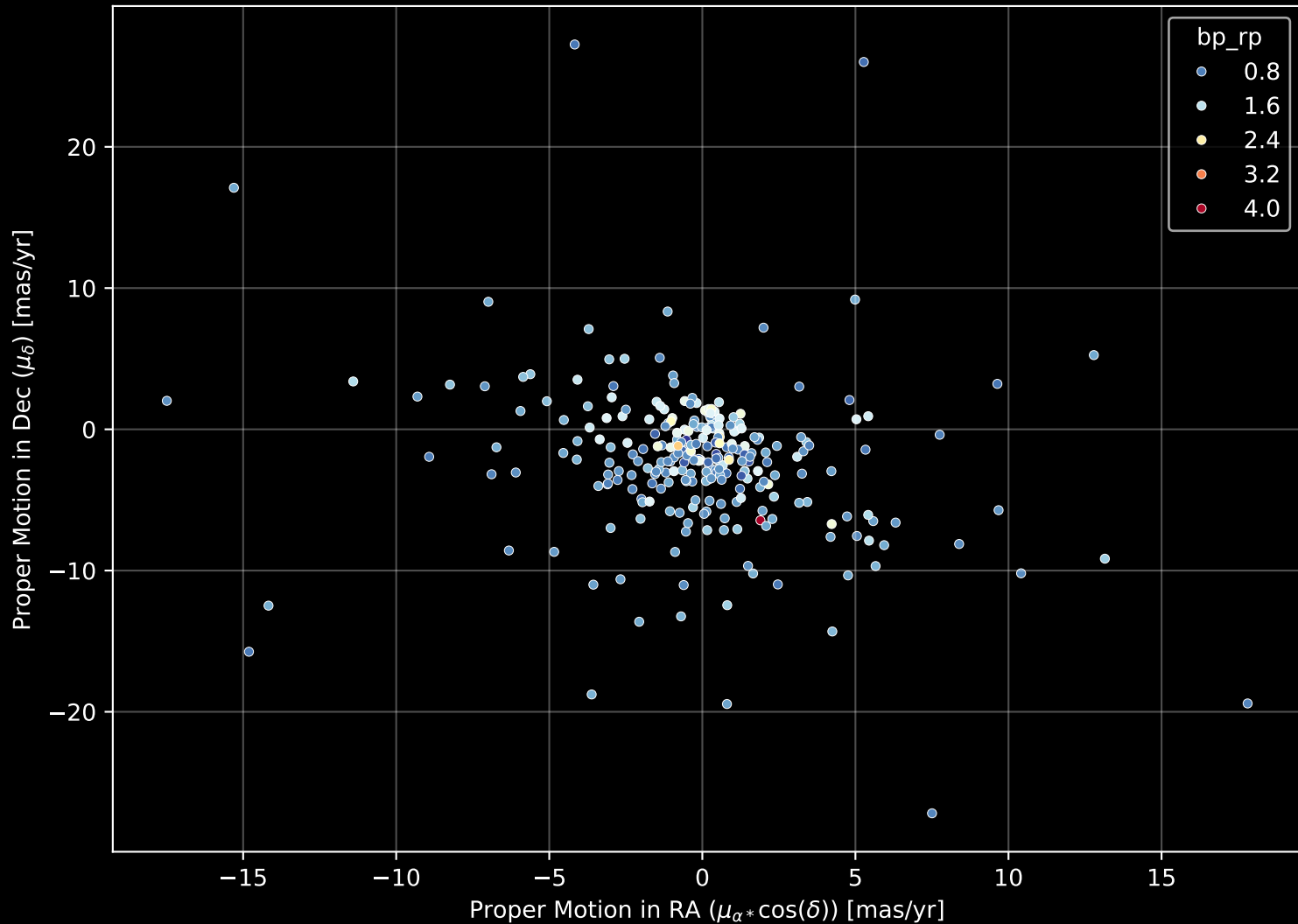
GALAH DR4 Field: [9274] Proper Motion Diagram (n= 270)
